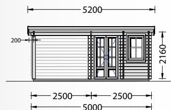
FACHADA NORTE
