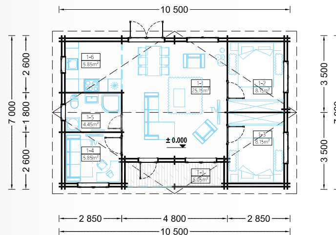
PLANTA BAIXA
