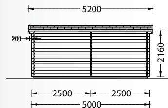
FACHADA SUL
