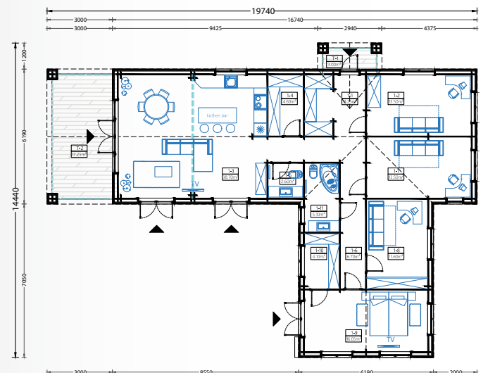
PLANTA BAIXA
