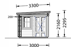
FACHADA LESTE
