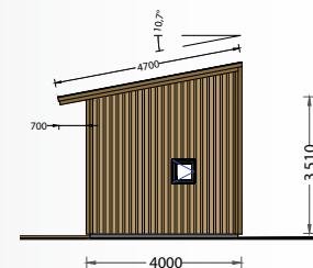
FACHADA SUL
