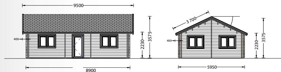
FACHADA SUL
