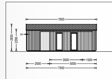
FACHADA NORTE
