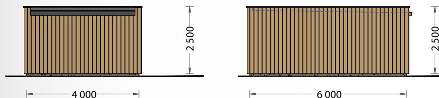
FACHADA SUL
