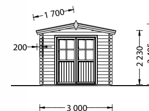
FACHADA LESTE
