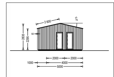
FACHADA OESTE
