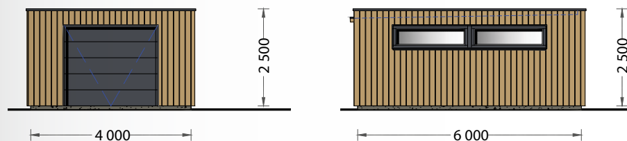
FACHADA NORTE
