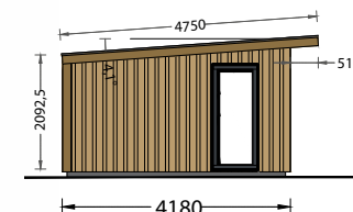
FACHADA LESTE
