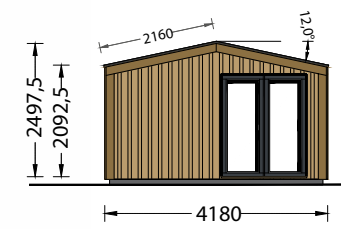
FACHADA LESTE
