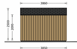
FACHADA LESTE
