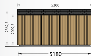
FACHADA SUL
