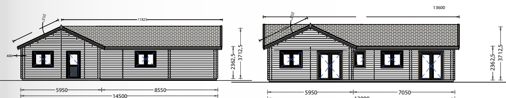
FACHADA NORTE
