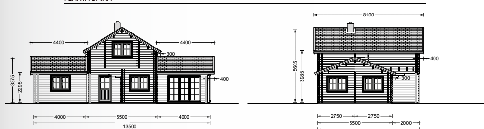
FACHADA NORTE
