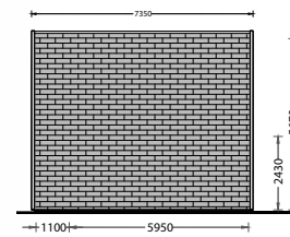
FACHADA LESTE
