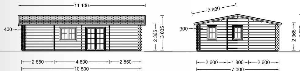
FACHADA SUL
