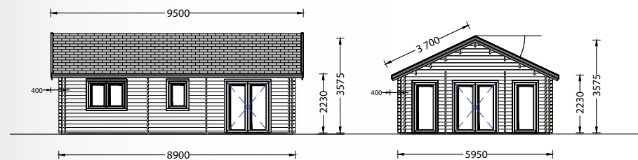
FACHADA NORTE
