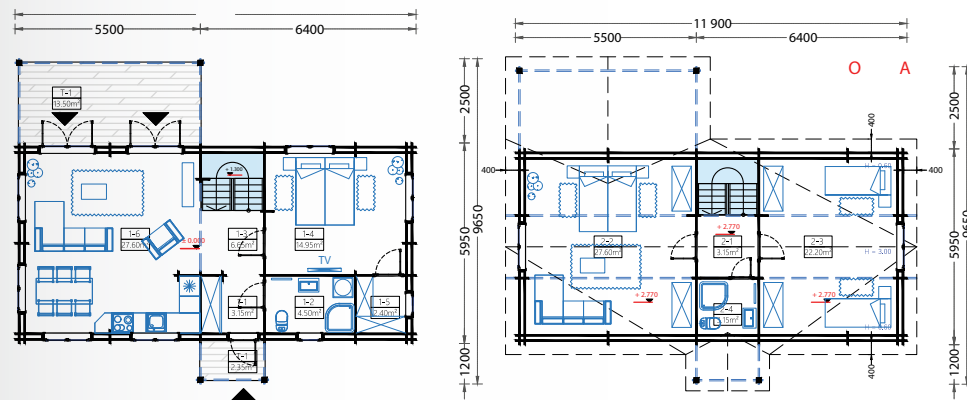
PLANTA BAIXA
