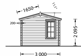
FACHADA OESTE
