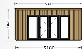
FACHADA NORTE
