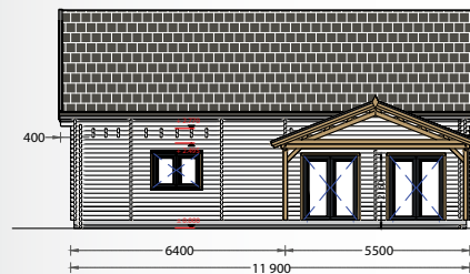
FACHADA SUL
