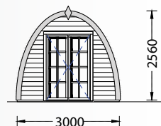
FACHADA NORTE
