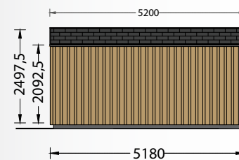
FACHADA SUL
