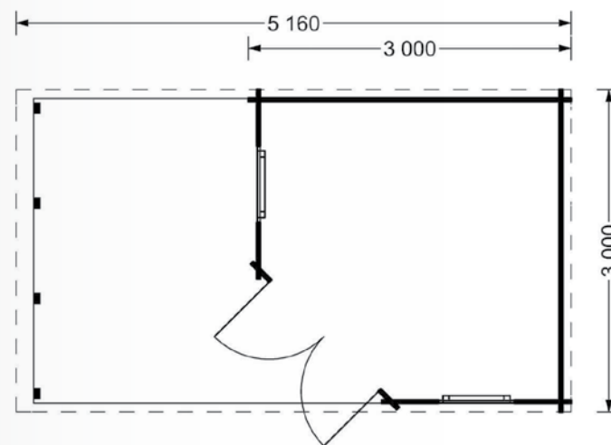
PLANTA BAIXA
