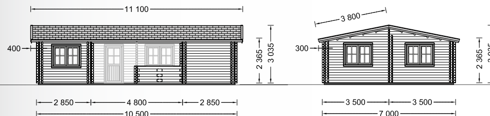
FACHADA NORTE
