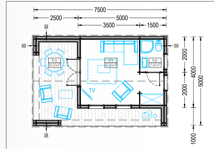
PLANTA BAIXA
