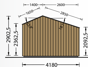
FACHADA SUL
