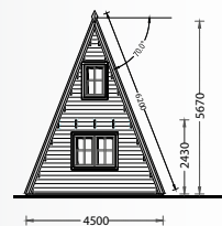
FACHADA SUL
