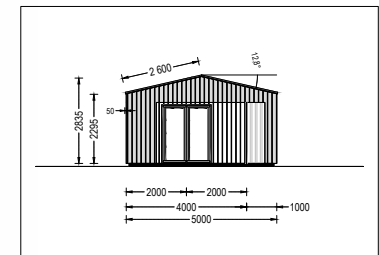
FACHADA LESTE
