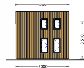
FACHADA OESTE
