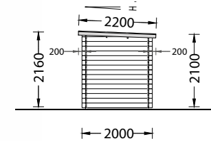
FACHADA OESTE
