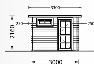
FACHADA NORTE
