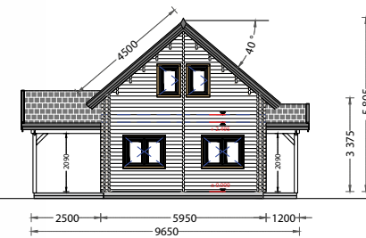
FACHADA LESTE
