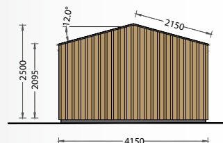
FACHADA SUL
