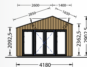
FACHADA NORTE
