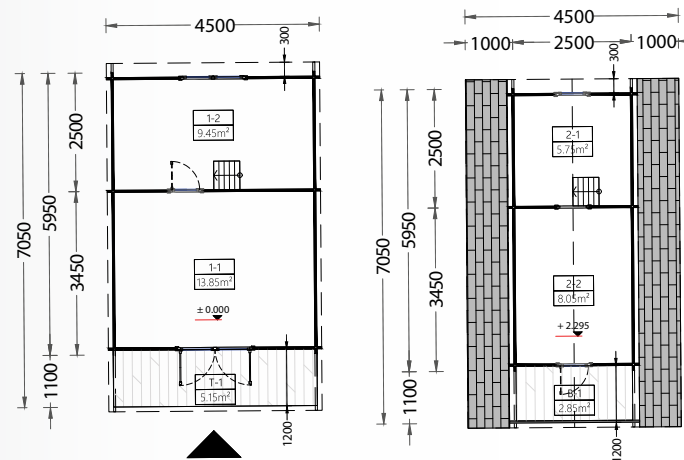
PLANTA BAIXA
