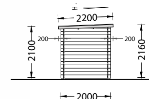
FACHADA LESTE
