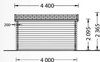
FACHADA SUL
