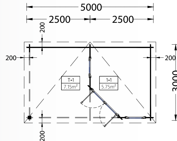
PLANTA BAIXA
