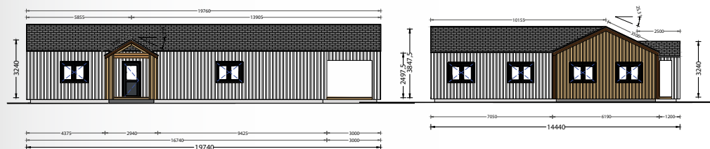
FACHADA SUL
