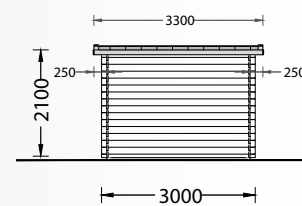
FACHADA SUL
