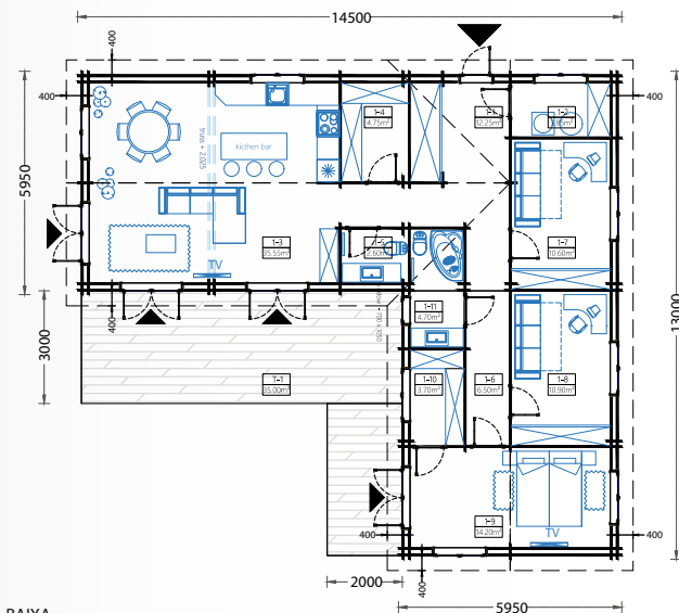
PLANTA BAIXA
