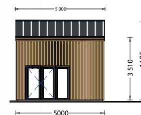
FACHADA LESTE
