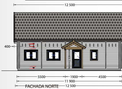
FACHADA NORTE
