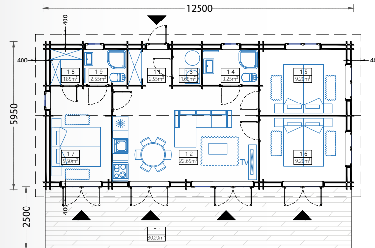
PLANTA BAIXA
