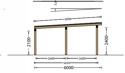
FACHADA OESTE
