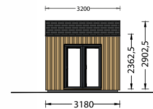
FACHADA OESTE
