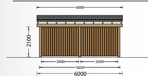
FACHADA SUL
