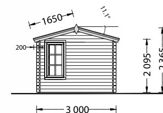
FACHADA LESTE
