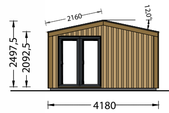
FACHADA OESTE
