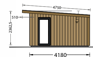
FACHADA OESTE
