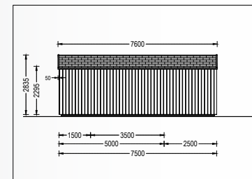
FACHADA SUL
