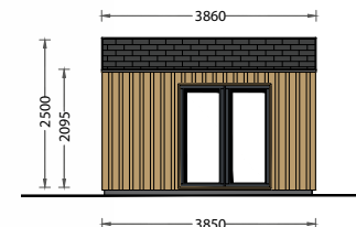
FACHADA OESTE
