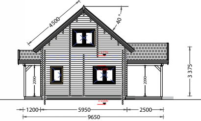
FACHADA OESTE
