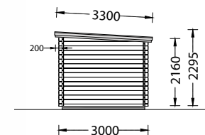
FACHADA OESTE
